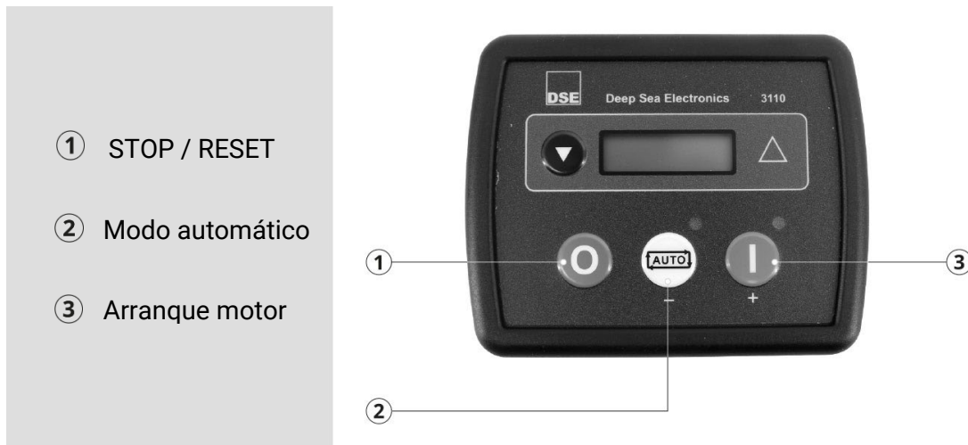
Imagen 12: Disposición modos de operación placa de control DSE 3110.
