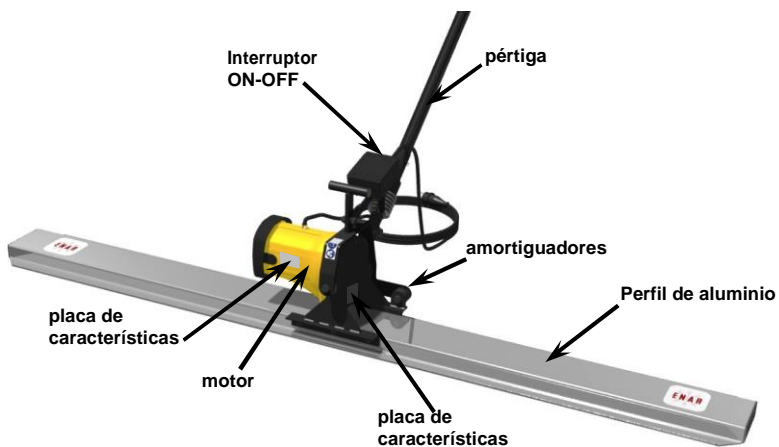
REGLAS VIBRO-EXTENEDORAS OSCILANTES CON MOTOR ELÉCTRICO O GASOLINA "QZ"
