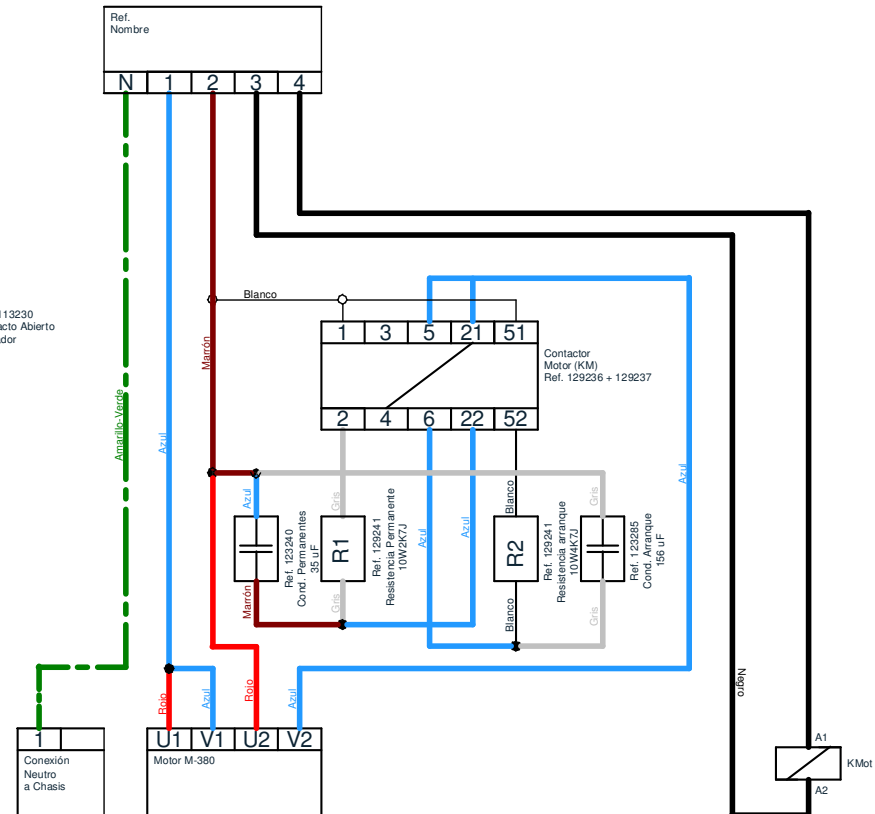
Plano 2 - Esquema Caja Condensadores
