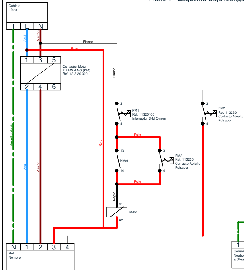
Plano 1 - Esquema Caja Mango
