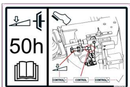
Fig. 53: Controlar el acoplamiento
