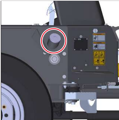
Fig. 226: Abertura de llenado de aceite hidráulico
