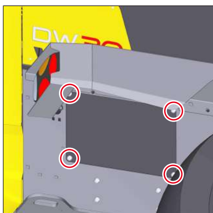
Fig. 220: Cubierta de mantenimiento 1
