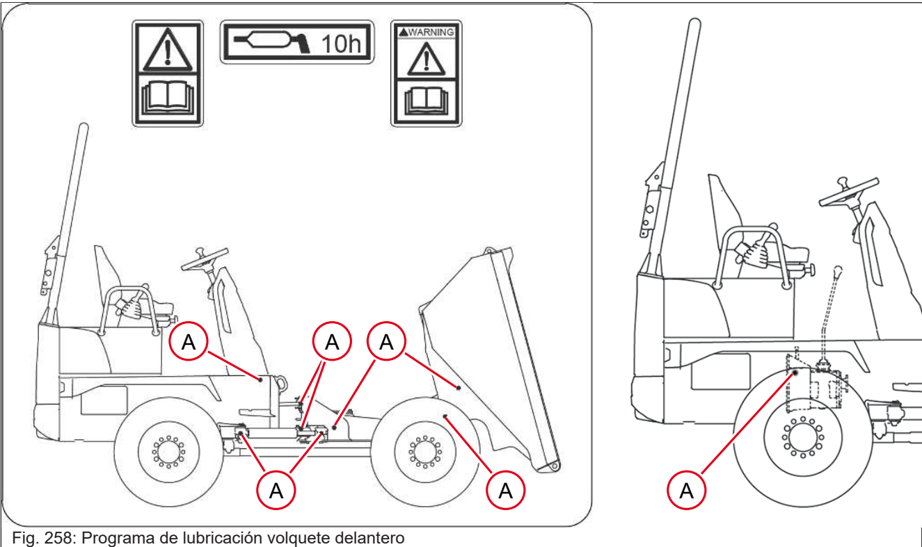
Fig. 258: Programa de lubricación volquete delantero
