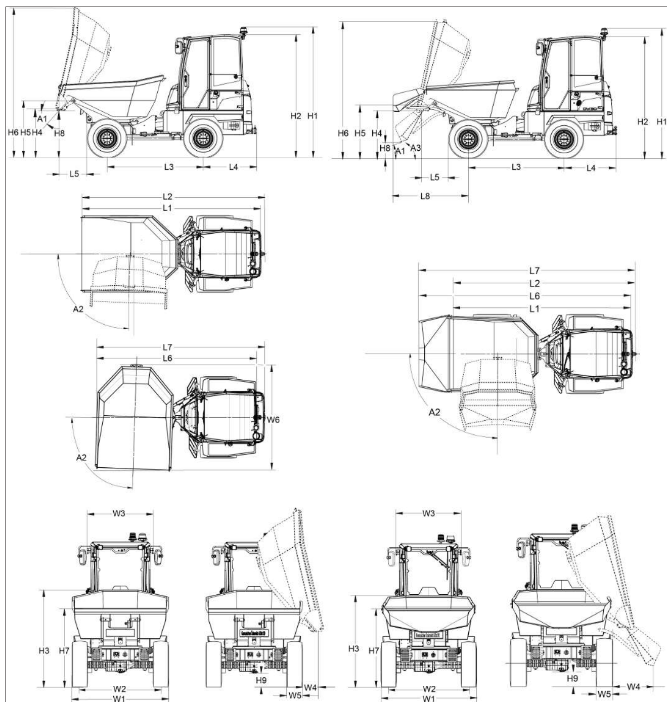
Fig. 299: Volquete giratorio, volquete para hormigón, cabina
