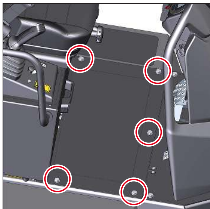
Fig. 195: Chapa de piso
