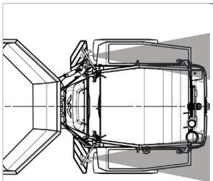
Fig. 88: Espejo retrovisor cabina (representación simbólica)
