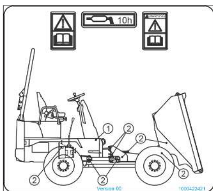
Fig. 51: Programa de lubricación
