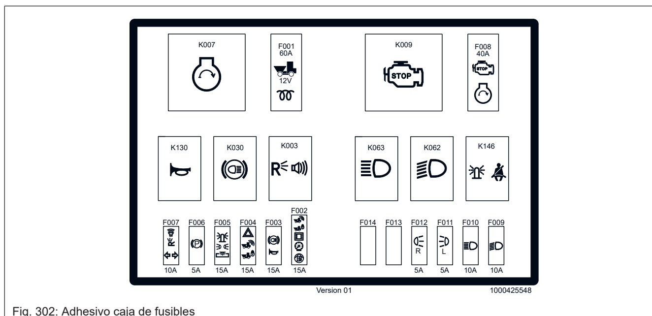
Fig. 302: Adhesivo caja de fusibles
