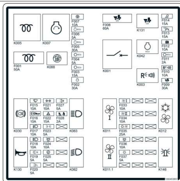
Fig. 304: Adhesivo, caja de fusibles variante 2
