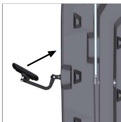
Fig. 103: Espejo del techo protector contra la intemperie
