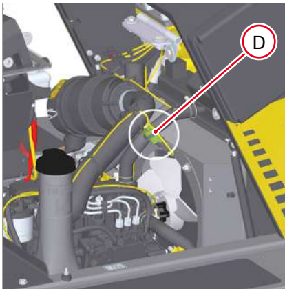
Fig. 279: Indicador del nivel de con- taminación 3TNV76
