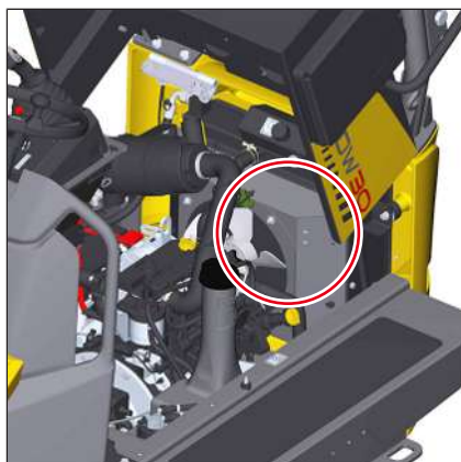
Fig. 283: Parte interior de la carcasa del ventilador
