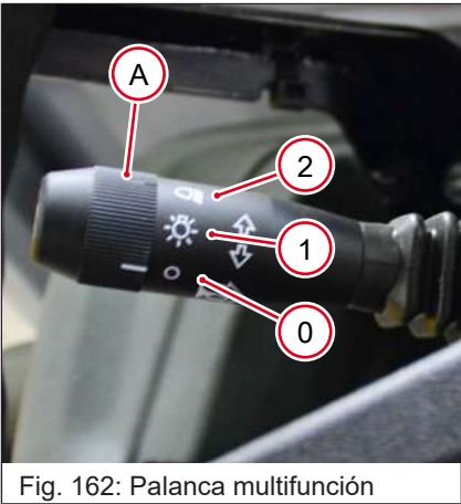
Fig. 162: Palanca multifunción
