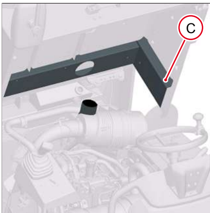
Fig. 278: Conducto de ventilación 403J-E17T
