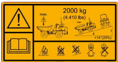
Fig. 23: Funcionamiento seguro
