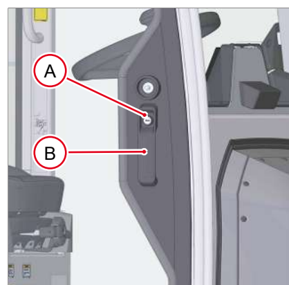
Fig. 76: Abrir y cerrar la puerta con llave
