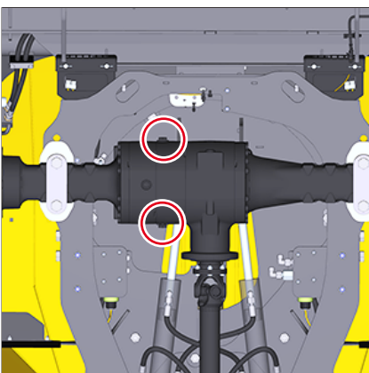
Fig. 200: Eje unidad de carga
