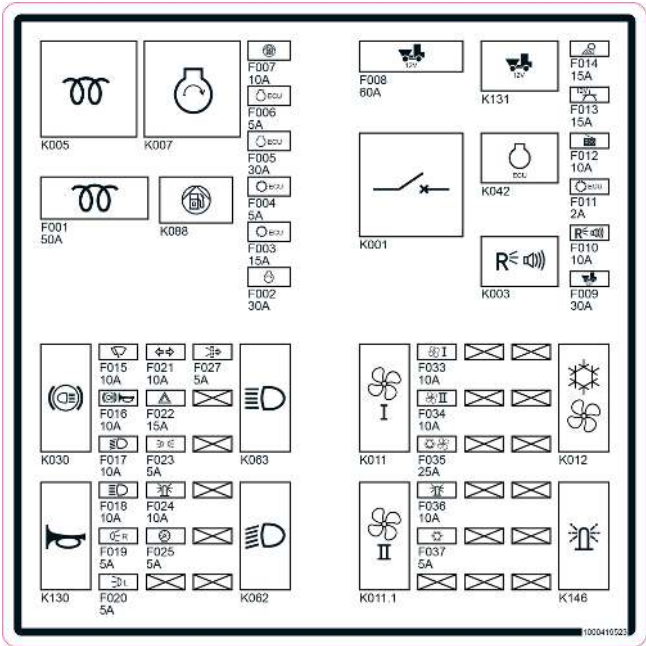
Fig. 303: Adhesivo, caja de fusibles variante 1
