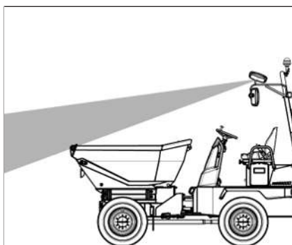
Fig. 90: Espejo para volquete de giro alto
