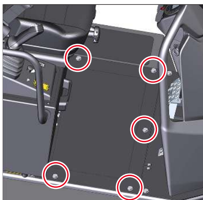
Fig. 192: Chapa de piso
