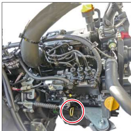
Fig. 239: 3TNV76 (DW20/DW30)
