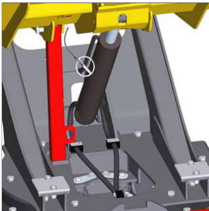
Fig. 261: Apoyo de mantenimiento montado
