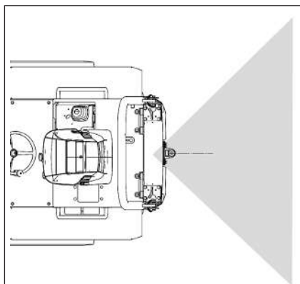
Fig. 93: Cámara 2 campo visual horizontal (representación simbólica)
