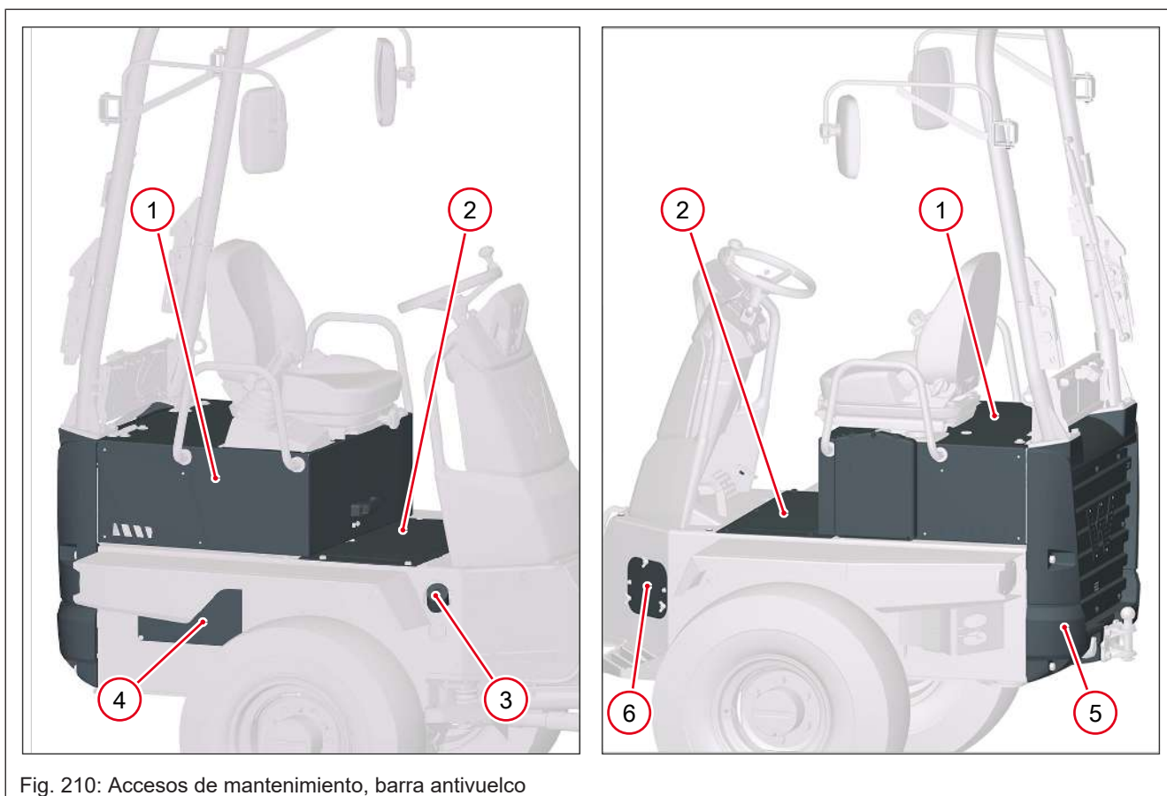
Fig. 210: Accesos de mantenimiento, barra antivuelco
