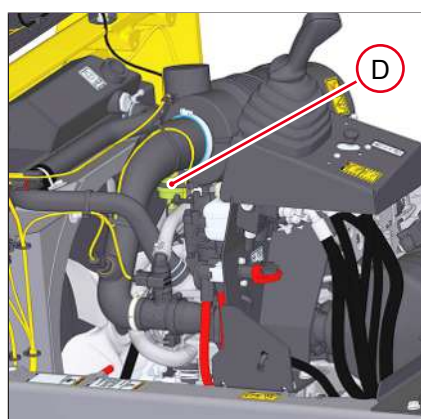
Fig. 281: Indicador del nivel de contaminación 403J-E17T
