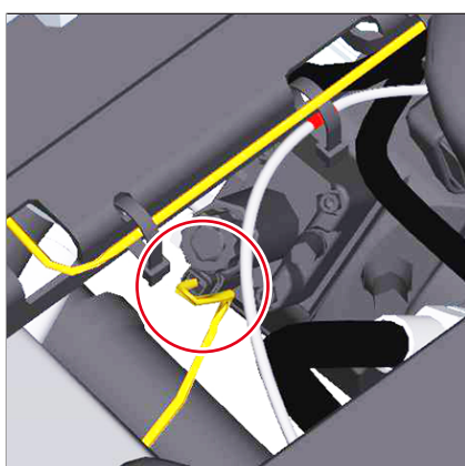
Fig. 194: Conector del motor de tracción
