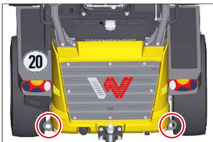
Fig. 207: Ojales de amarre de la unidad de accionamiento
