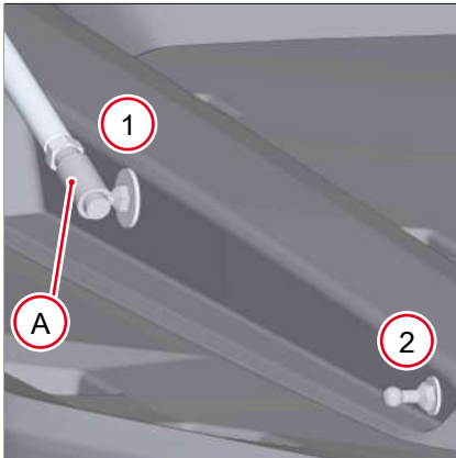
Fig. 104: Bloqueos del techo protector contra la intemperie a la izquierda
