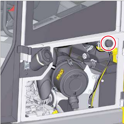
Fig. 251: Abertura de llenado del agente refrigerante, cabina
