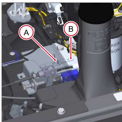
Fig. 287: Posición de la herramienta de medición
