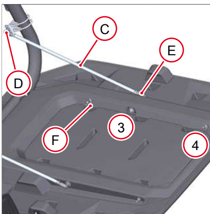
Fig. 105: Bloqueos del techo protector contra la intemperie a la derecha
