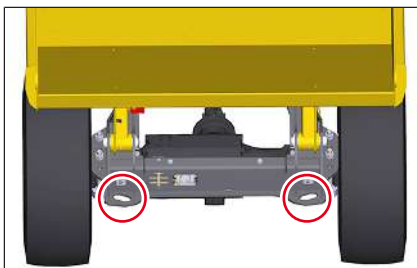
Fig. 208: Cánkamos de amarre de la unidad de carga
