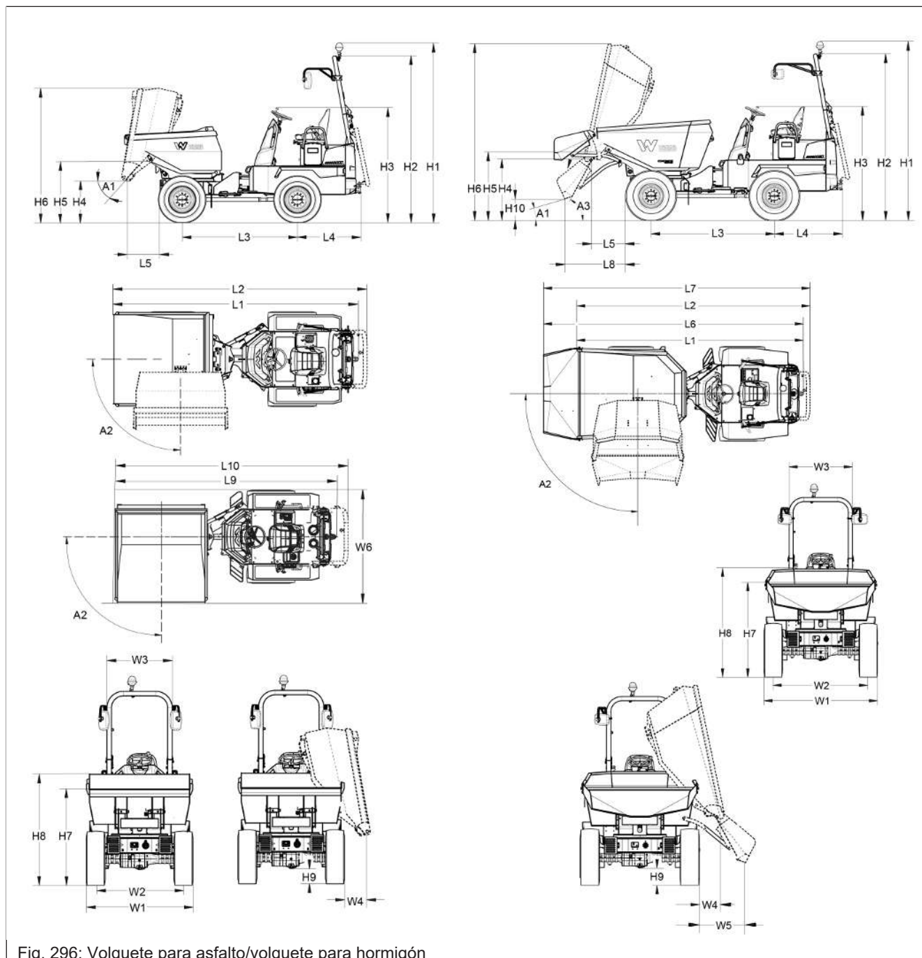
Fig. 296: Volquete para asfalto/volquete para hormigón
