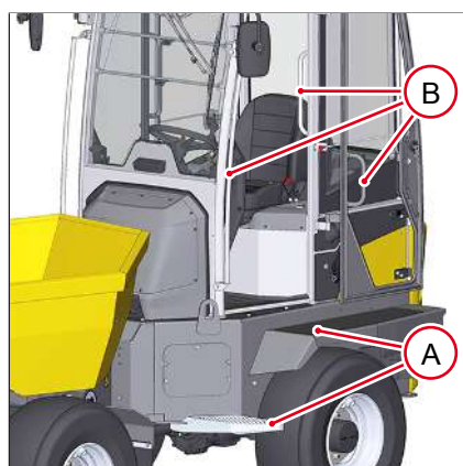
Fig. 75: Subir y bajar, cabina
