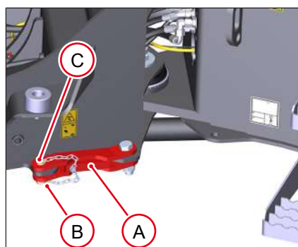
Fig. 203: Bloqueo articulado desmontado
