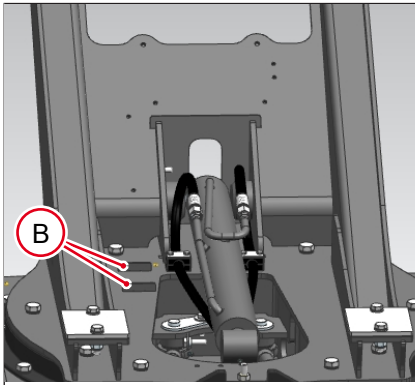
Fig. 260: Placas delimitadoras
