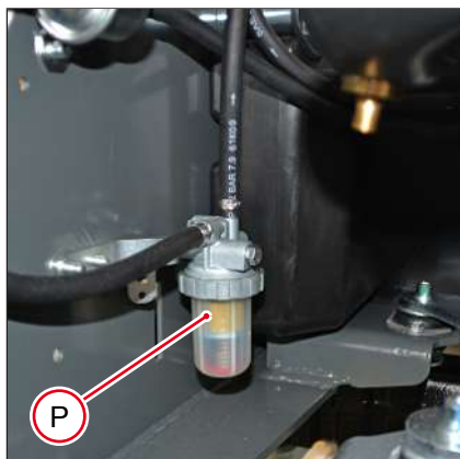
Fig. 229: Prefiltro 3TNV76, 3TNV88
