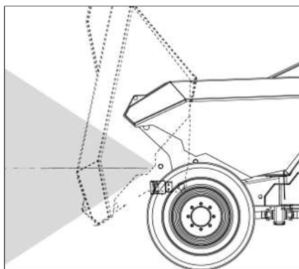
Fig. 92: Cámara 1 campo visual vertical (representación simbólica)
