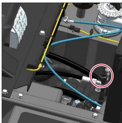
Fig. 197: Válvula limitadora de presión superior
