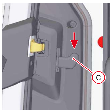
Fig. 77: Abrir la puerta desde adentro
