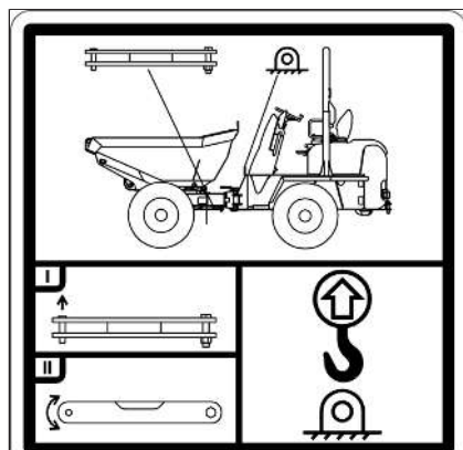
Fig. 42: Carga con grúa
