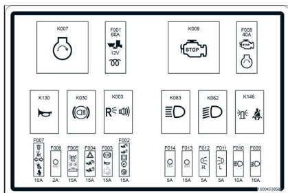
Fig. 50: Fusibles y relés
