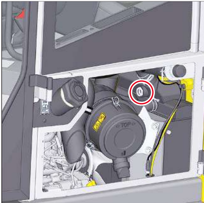
Fig. 248: Comprobar el nivel de agente refrigerante, cabina
