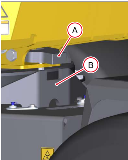
Fig. 180: Desbloquear el volquete
