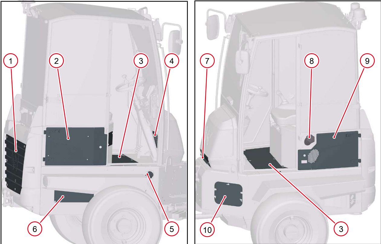
Fig. 211: Accesos de mantenimiento cabina
